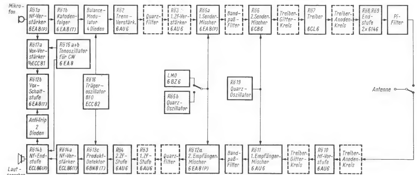
Bild 2. Das Blockschaltbild des Gerätes SB 100
