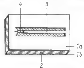
Bild 1. Prinzip eines elektronisch abstimmbaren Leitungskreises aus doppelseitig mit leitender Folie kaschiertem Dielektrikum (Erklärung der Einzelheiten im Text)
