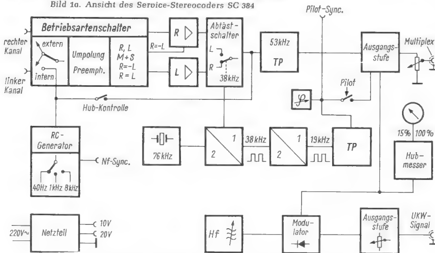
Bild 1b. Prinzipschaltbild des Stereocoders von Nordmende
