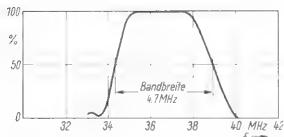
Bild 4a. Zf-Durchlaßkurve, linear dargestellt
