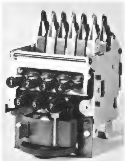
Bild 2. Tastenaggregat des Monomat-Electronic in den Fernsehempfängern der Europa-Klasse von Grundig
