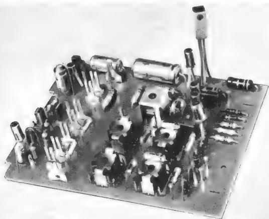
Bild 10. Decoderträgerplatte, links Vorverstärker, daneben die Haltefedern für den Decoder, im Vordergrund das LC-Filter, rechts im Hintergrund der Schwell- und Anzeigeverstärker
