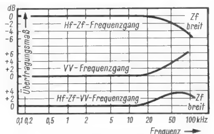
Bild 2. Frequenzgang des Zf-Verstärkers, Bandbreiteschalter auf breit (oben); Frequenzgang des Vorverstärkers (Mitte); Frequenzgang mit angeschaltetem Vorverstärker (unten)
