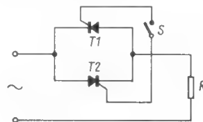
Antiparallelschaltete Thyristoren zum Steuern einer Wechselstromleistung. Der Schalter S braucht nur einen Bruchteil der Schaltleistung der Thyristoren aufzuweisen. Er kann auch durch einen Halbleiter dargestellt werden
