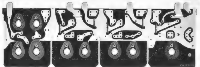
Bild 2. Druckplatte des Zf-Verstärkers
