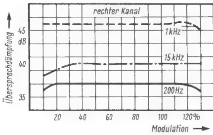
Bild 14. Übersprechdämpfung als Funktion des Modulationsgrades
