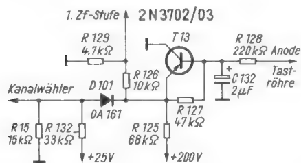
Bild 5. Schaltung der Impedanzwandlerstufe der Regelung
