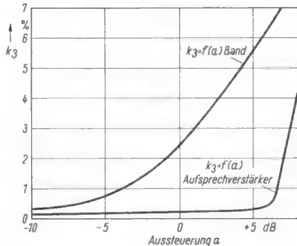
Bild 4. Verlauf des Klirrfaktors k_3 in Abhängigkeit vom Aussteuerungsgrad a (Band). Verlauf des Klirrfaktors des Aufsprecherstärkers in Abhängigkeit von dessen Aussteuerungsgrad. Der Klirrfaktor des Aufsprecherstärkers liegt bei Vollaussteuerung bei 0,25 % (Band: Normcharge 110 211, BASF; Gerät: Klasse 19 Hi-Fi, Uher-22-Spezial; v = 19,05 cm/sec; N_f = 333 Hz; Aussteuerung: 0 dB = 200 mV)
