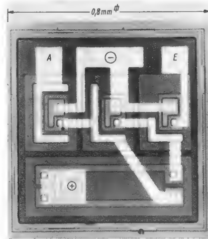
Bild 14. Integrierter Schaltkreis OM 200 mit drei Transistoren und zwei Widerständen auf einer Fläche von weniger als 1 mm 2 (Valvo)
