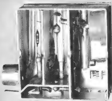
Bild 4. Aufbau eines zweistufigen UHF-Steckverstärkers
