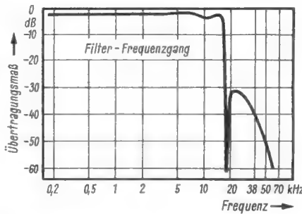
Bild 5. Frequenzgang des Filters gem. Bild 4
