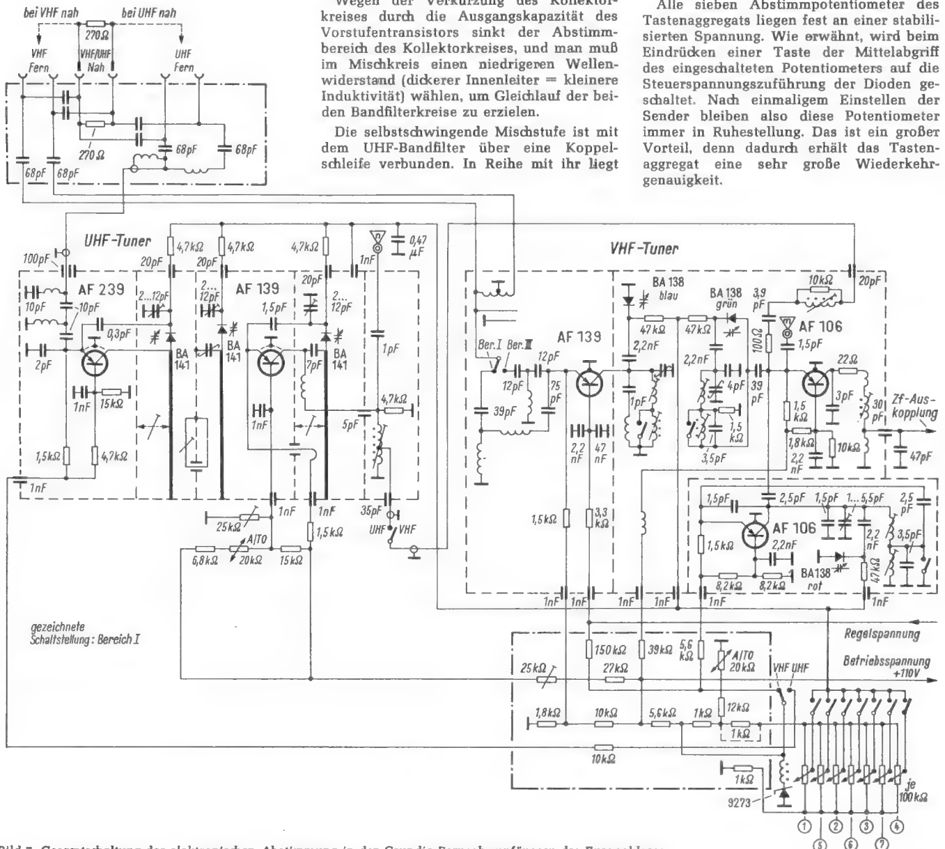
Bild 7. Gesamtschaltung der elektronischen Abstimmung in den Grundig-Fernsehempfängern der Europaklasse
