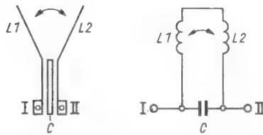
Bild 6. Schaltung eines Parallelkreises und Darstellung der Variospule
