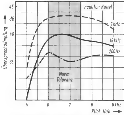
Bild 15. Übersprechdämpfung in Abhängigkeit vom Hub der Pilotfrequenz
