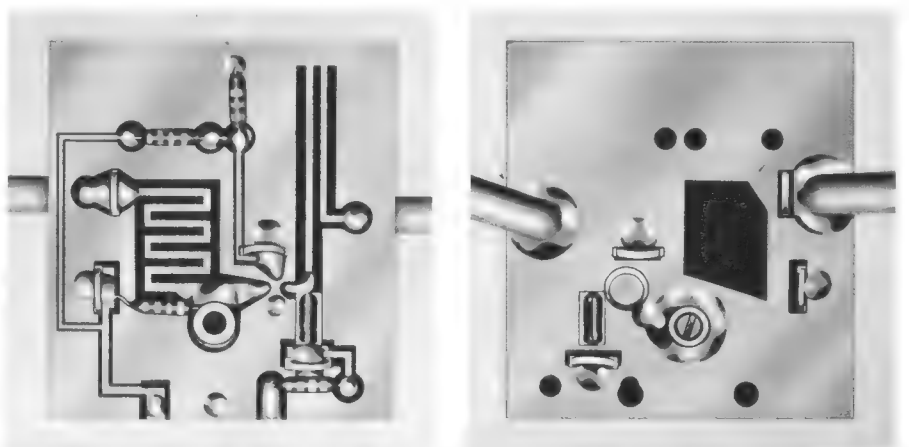
Bild 3. Draufsicht (links) und Rückansicht (rechts) des einstufigen UHF-Verstärkers nach Bild 2 in natürlicher Größe
