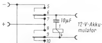
Bild 1. Prinzip der Polumschaltung mit einem polarisierten Relais
