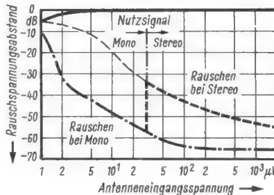
Bild 7. Rauschverhältnis bei Mono- und Stereoempfang
