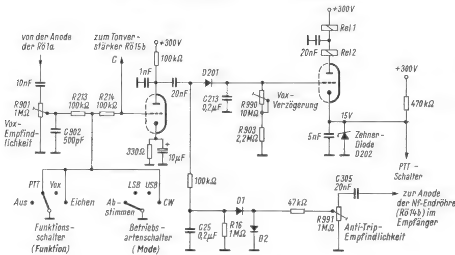
Bild 3. Vox- und Anti-Trip
