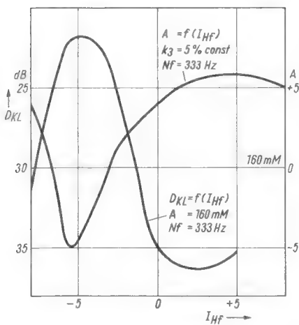
Links: Bild 3. Abhängigkeit der Aussteuerfähigkeit A eines Tonbandes vom Hochfrequenz-Vormagnetisierungsstrom I_{HF} und Abhängigkeit der Klirrdämpfung D_{KL} von dem Hochfrequenz-Vormagnetisierungsstrom I_{HF} . Band: LGS 26, Normcharge 110 211, v = 9,53 cm/sec (nach Unterlagen der BASF)
