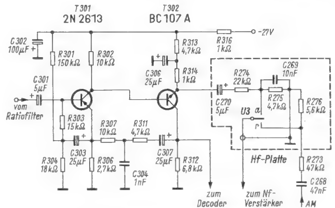
Bild 1. Schaltung des Vorverstärkers
