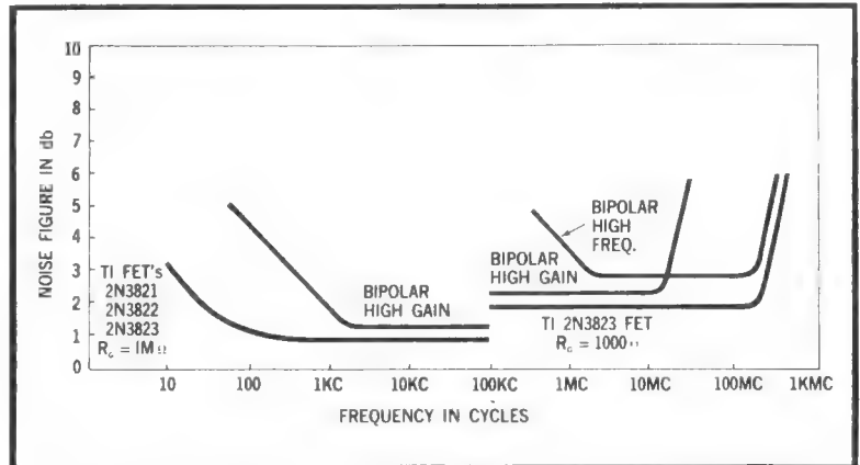
Abb. 6 - Optimale Rauschzahl des TI 2N3823 FET im Vergleich mit weitverbreiteten bipolaren Transistoren.
