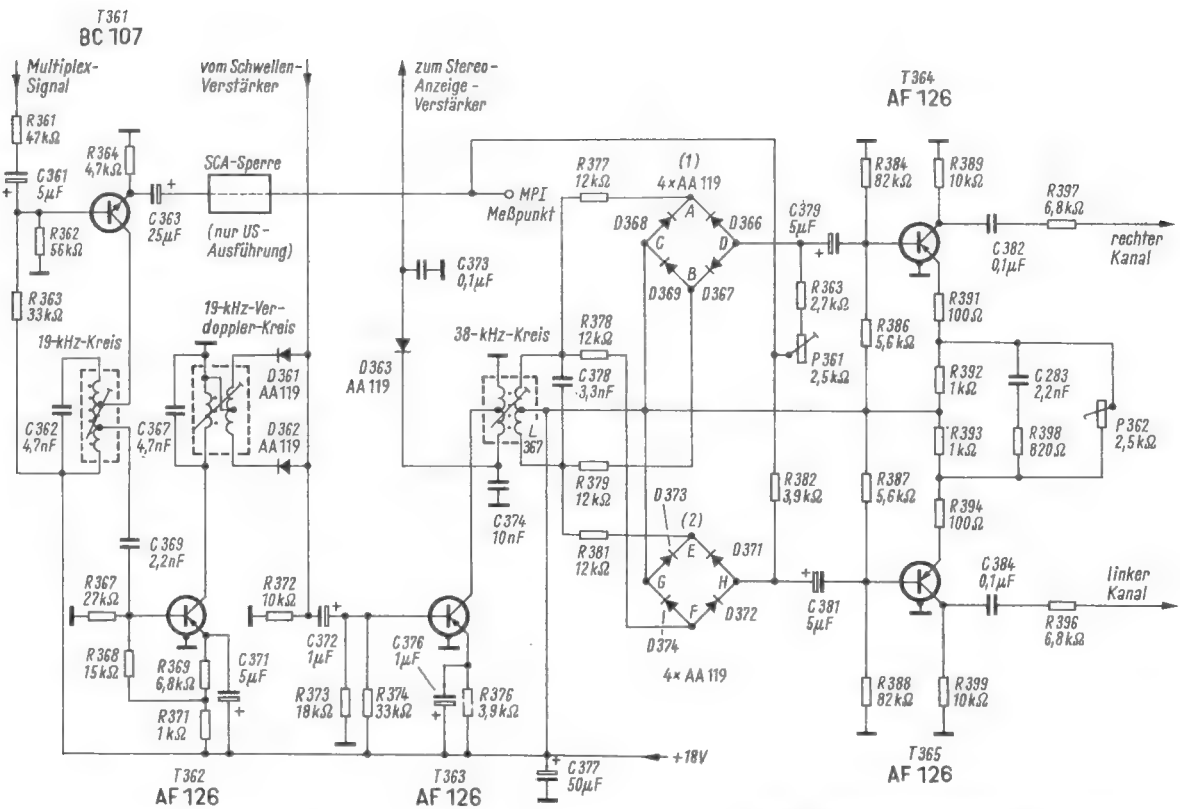
Bild 3. Schaltung des Decoders
