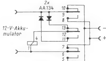
Bild 2. Polumschaltung mit Relais und Dioden
