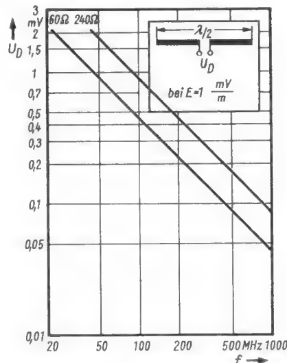
Abhängigkeit der Empfangsspannung von der Frequenz bei gegebener Feldstärke
