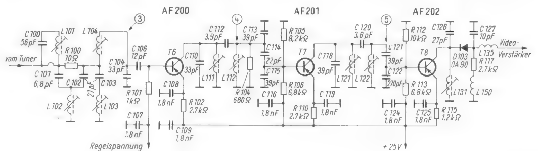
Bild 3. Schaltung des Zf-Verstärkers
