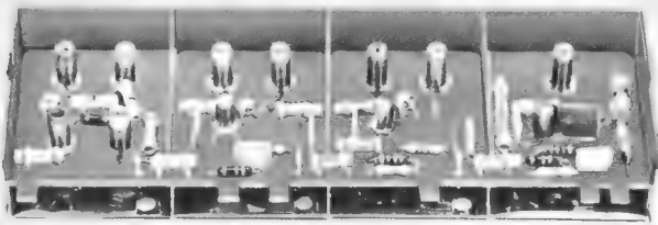
Bild 1. Der Zf-Verstärker mit den vier Kammern und abgenommenem Deckel
