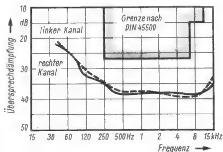
Bild 12. Übersprechdämpfung des Decoders, über den Hf-Teil gemessen
