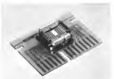
Fassung für Halbleiterschaltkreise in Flachpackform von Texas Instruments. Die eigentliche Schaltstufe ist das kleine helle Plättchen
