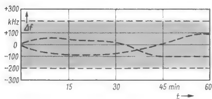
Bild 8. Temperaturgang, gültig für alle UHF-Kanäle (Toleranzfeld und zwei gemessene Kurven)
