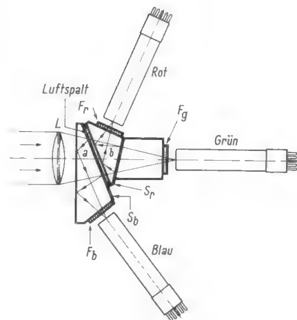
Bild 4. Strahlengang durch den Farbzerlegungsblock. L = Kameraobjektiv; F_r , F_g , F_b = Rot-, Grün-, Blau-Korrekturfilter; S_r , S_b = rot- bzw. blaureflectierende Schicht
