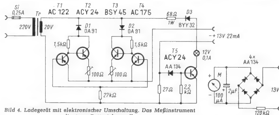
Bild 4. Ladegerät mit elektronischer Umschaltung. Das Meßinstrument dient zur Batteriekontrolle
