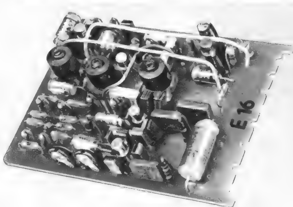
Bild 11. Die Stereodecoder-Platine hat vergoldete Kontaktbahnen, die in die Haltefedern (Bild 10) eingeschoben werden
