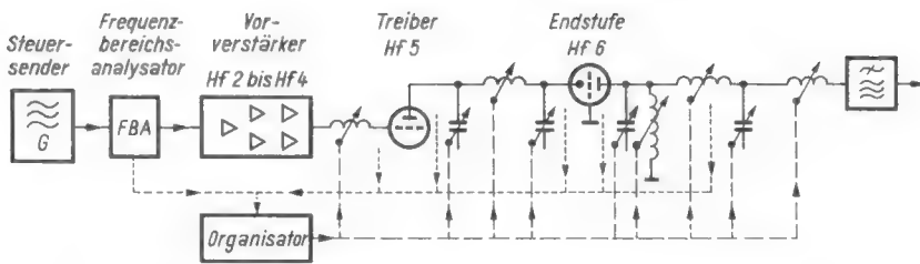
Bild 3. Prinzip des Hochfrequenzteils mit Abstimmung durch den Organisator
