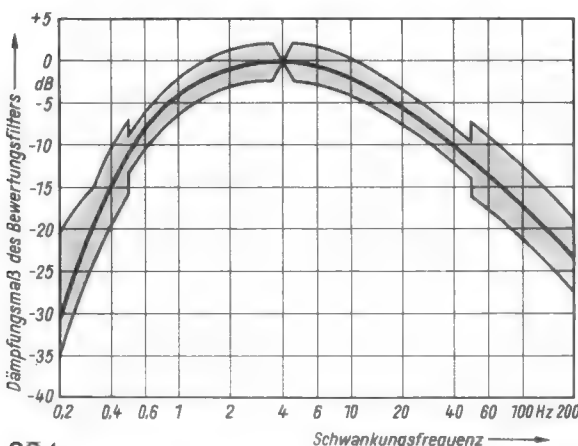
Links: Bild 1. Bewertungskurve nach DIN 45 507 mit Toleranzbereich
