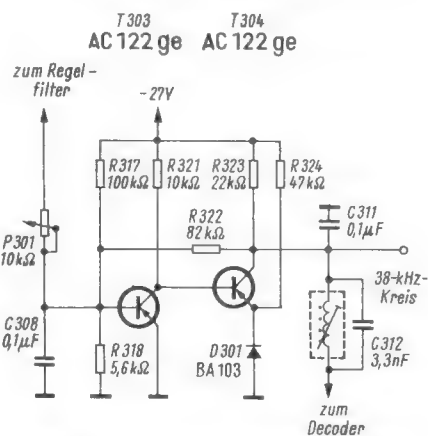
Bild 9. Schaltung des Schwellenverstärkers
