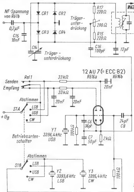
Links: Bild 4. Balancemodulator und Trägeroszillator
