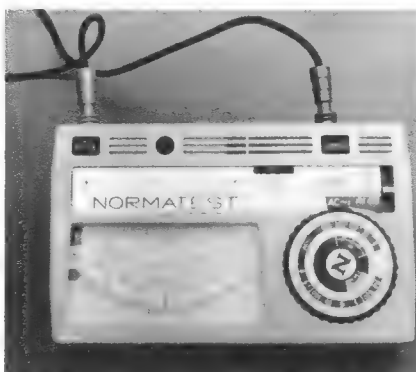
Leichter und handlicher Vielfachmesser Normatest; die Spezialmeßleitungen sitzen so fest, daß man das Gerät an den Schnüren hängend benutzen kann; für die Prüfgriffe gibt es noch aufsteckbare Verlängerungsspitzen
