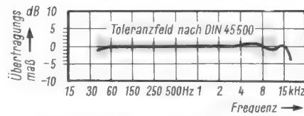
Bild 16. Frequenzgang am Filterausgang, über den Hf-Teil gemessen
