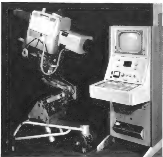
Bild 3. Die Kamera auf Gully-Stationwagen; rechts das Kontrollgestell mit offenem Bedienpult und ausgeschwenktem Kontrollpanel für den Speisungs- und Stabilisierungsteil
