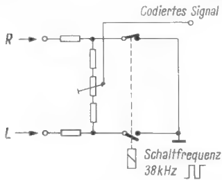
Bild 3. Das Arbeitsprinzip des nach dem Kurzschlußverfahren arbeitenden Abtastschalters
