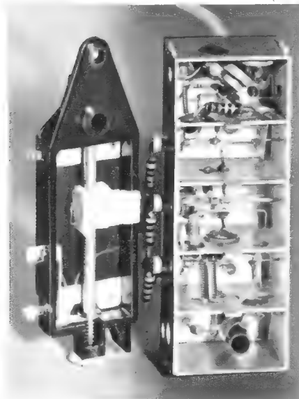
Bild 3. UHF-Diodentuner und ein Abstimmpotentiometer des Monomat-Electronic. Der UHF-Tuner hat die Abmessungen 76 mm x 28 mm x 24 mm
