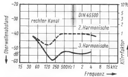
Bild 17. Oberwellenabstand als Funktion der Frequenz, gemessen bei (40 + 7,5) kHz Hub am Decoderausgang
