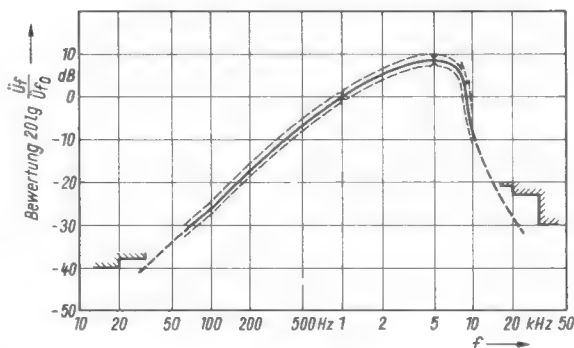
Rechts: Bild 5. Bewertungskurve nach DIN 45 405 für die Spitzenwertspannung von Geräuschspannungen. Die unterbrochenen Linien begrenzen das Toleranzfeld. Bei niedrigen und hohen Frequenzen setzt sich die Kurve unterhalb des schraffierten Bereiches fort
