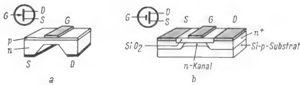
Bild 12. Schematischer Aufbau von Feldeffekttransistoren. a = Germanium-Sperrschicht-Typ, b = Silizium-Planar-MOS-Typ. (G = Gate oder Tor \triangle Gitter, S = Source oder Quelle \triangle Katode, D = Drain oder Abfluß \triangle Anode)
