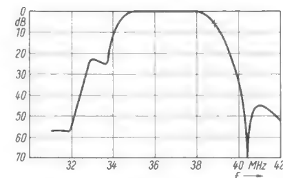
Bild 4b. Die Zf-Durchlaßkurve im logarithmischen Maßstab dargestellt. Die tiefe Einsattelung bei 40,4 MHz wird durch die Nachbartonfalle erzielt
