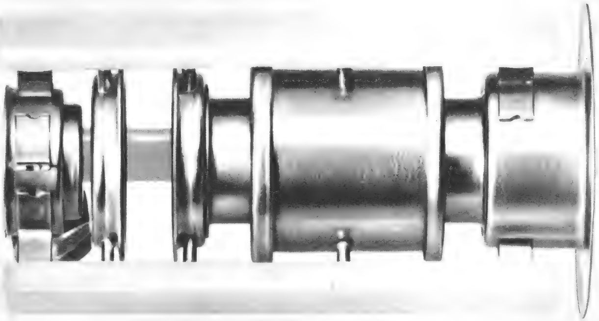
Elektronenoptik der SEL-Bildröhre, 3,5fach vergrößert
