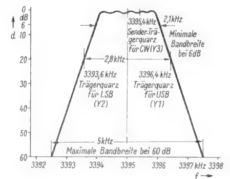
Bild 5. Durchlaßkurve des Quarzfilters mit Trägerfrequenzen
