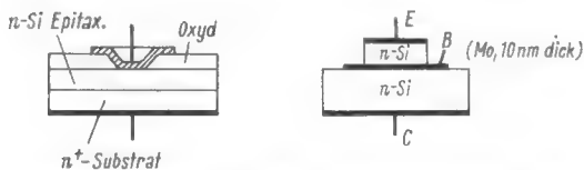
Bild 10. Schematischer Aufbau einer Schottky-Diode (links) und eines Metallbasis-Transistors (rechts)
