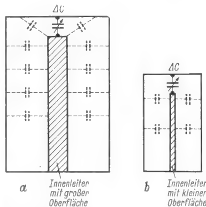
Bild 5a. Topfkreis mit großer Oberfläche des Innenleiters; dadurch viel Streukapazität (hoher Kapazitätsbelag), kleine Induktivität, kleiner Wellenwiderstand, große Topfabmessungen. Für ein bestimmtes Abstimmfrequenzverhältnis ist ein großer Betrag von \Delta C erforderlich
