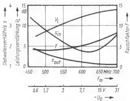
Bild 4. Meßwerte des beschriebenen Verstärkers: Leistungserhöhung, Rauschfaktor und Stehwellenverhältnis als Funktion der Bandmittenfrequenz bzw. der Diodenspannung
