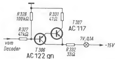
Bild 8. Schaltung des Anzeigeverstärkers
