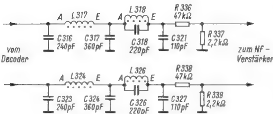
Bild 4. Schaltung des LC-Filters
