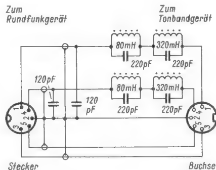
Schaltung einer Überspielleitung für Tonbandaufnahmen zum Abriegeln der Hilfsfrequenzen 19 kHz und 38 kHz, die beim Rundfunk-Stereoeempfang auftreten
