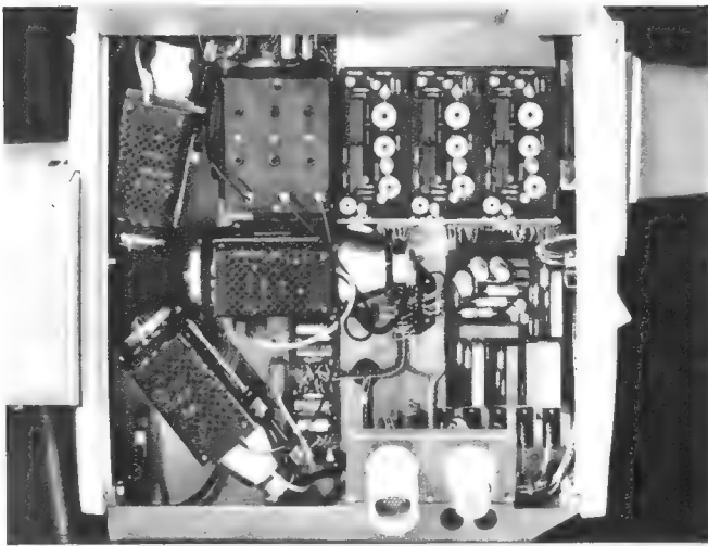
Bild 5. Innerer der Kamera mit Farbzerlegungsblock im Zentrum der drei Aufnahmeröhren (links) und dem gesamten elektronischen Teil, bei nach oben aufgeklappter linker Seitenwand
