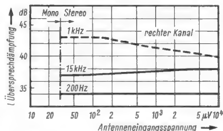
Bild 13. Übersprechdämpfung in Abhängigkeit von der Antenneneingangsspannung
