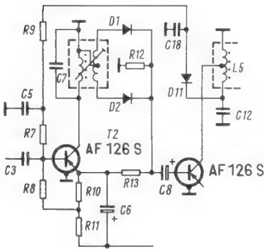
Bild 6. Schaltungsausschnitt vom Decoder mit Schwelle
