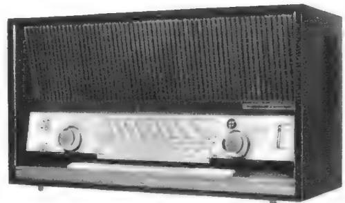
Tannhäuser-Stereo, 4 Wellenbereiche, UKW-Scharfabstimmung, 17 Watt Ausgangsleistung
