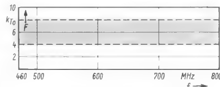
Bild 6. Toleranzfeld der Rauschzahl des UHF-Diodentuners
