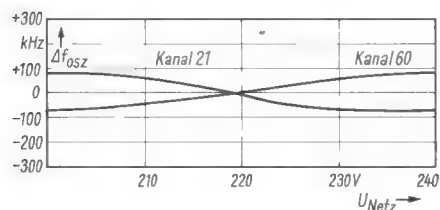
Bild 9. Änderung der Oszillatorfrequenz in Abhängigkeit von Schwankungen der Netzspannung
