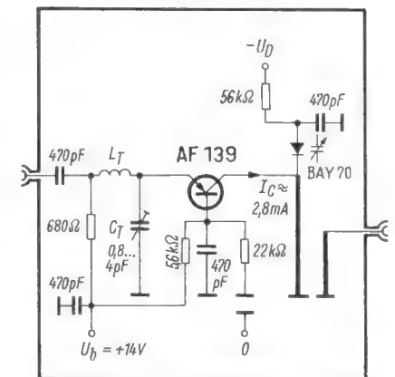
Bild 2. Schaltbild eines einstufigen UHF-Verstärkers mit Diodenabstimmung
