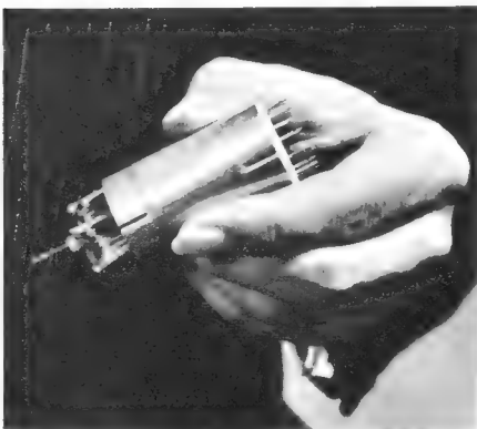
In dem Siemens-Gleichstrommotor sind dem Verschleiß unterliegende Teile für die Drehzahlregelung durch Transistoren, Widerstände, Dioden und Hallgeneratoren ersetzt
