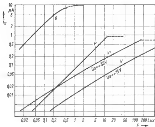
Links: Bild 1. Durchschnittswerte der i_g/E -Kennlinien für Super-Orthikon (O), Plumbikon (P) und zwei verschieden empfindlich eingestellte Vidikons (V und V'). Im doppellogarithmischen Maßstab kommt die Krümmung der Kennlinien nur durch ihre geringe Steilheit zum Ausdruck
